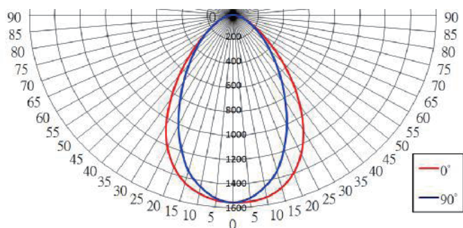
照度分布図
