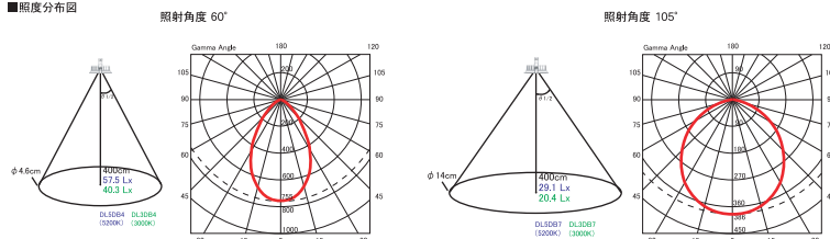
■照度分布図
